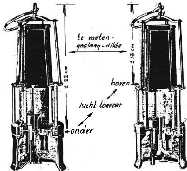
Veiligheidslamp met dubbele gaaskap
